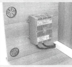
Fig.2 - INSTALLAZIONE VERTICALE
