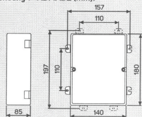
Abbildung 1 - ABMABE (mm):
